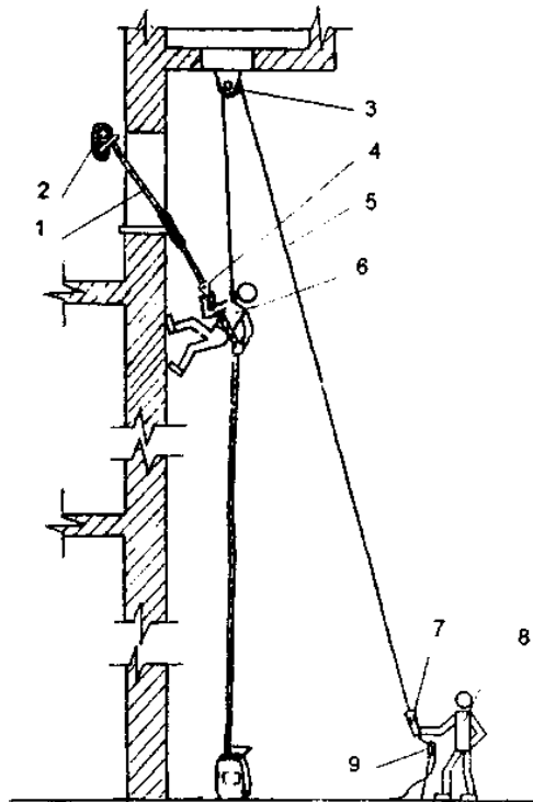
Рисунок 4. Схема страховки при спуске испытателей на УКСП: 1 - канат УКСП; 2 - силовой элемент объекта или испытательного стенда; 3 - блок; 4 - тормозное устройство; 5 - страховочная веревка; 6 - испытатель; 7 - приспособление для экстренного заклинивания веревки; 8 - оператор, осуществляющий страховку испытателя; 9 - якорь
