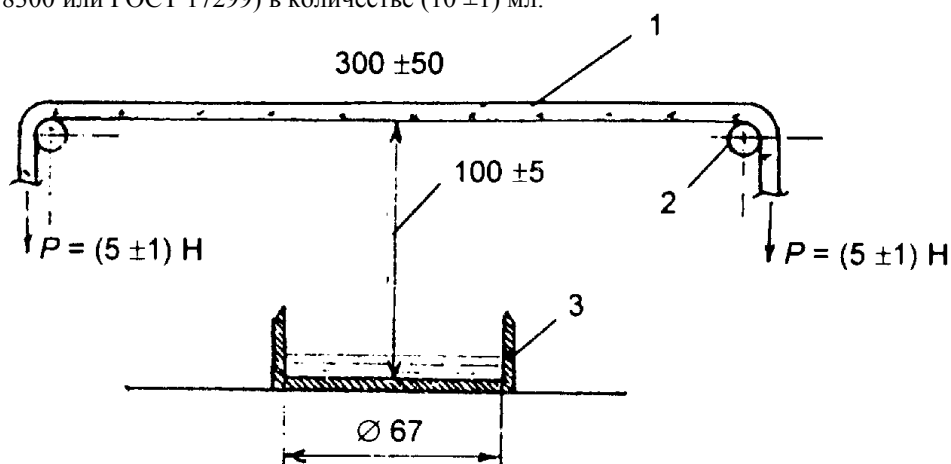
Рисунок 6. Схема станда для испытания каната УКСП на воздействие открытого пламени:
