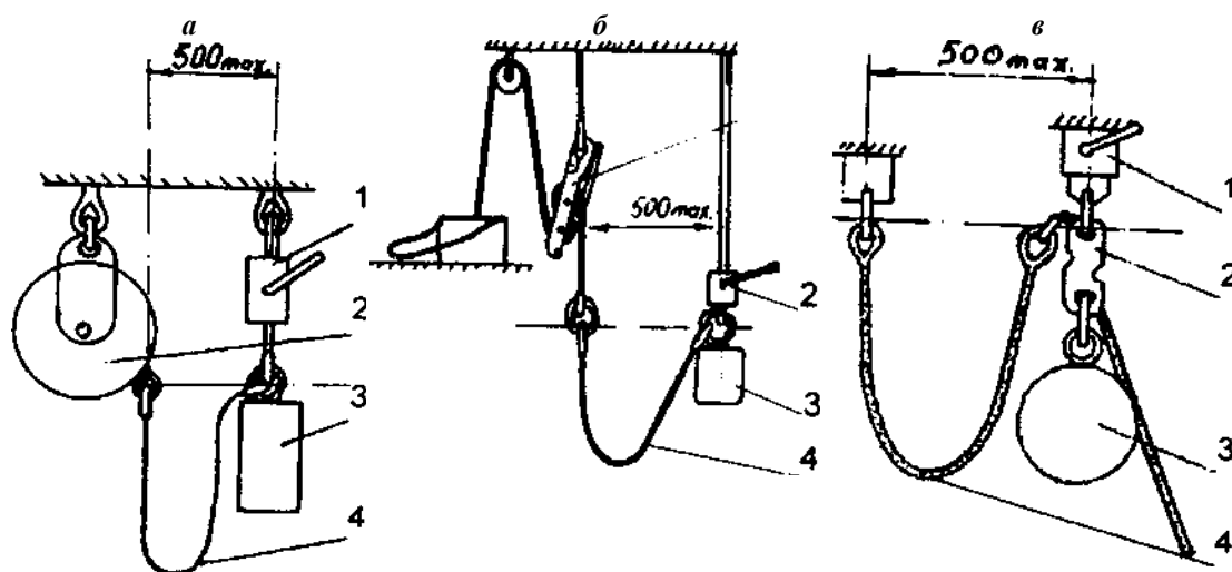
Рисунок 5. Схемы испытания УКСП на динамическую прочность:
